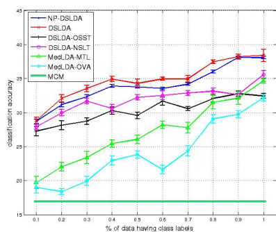
Fig. 1. p_1 = 0.5 (aYahoo)
